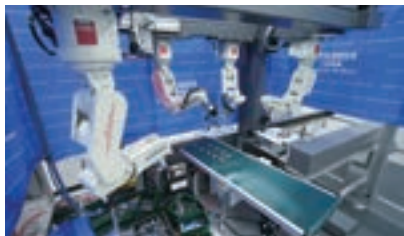
部品整列ロボットシステム
